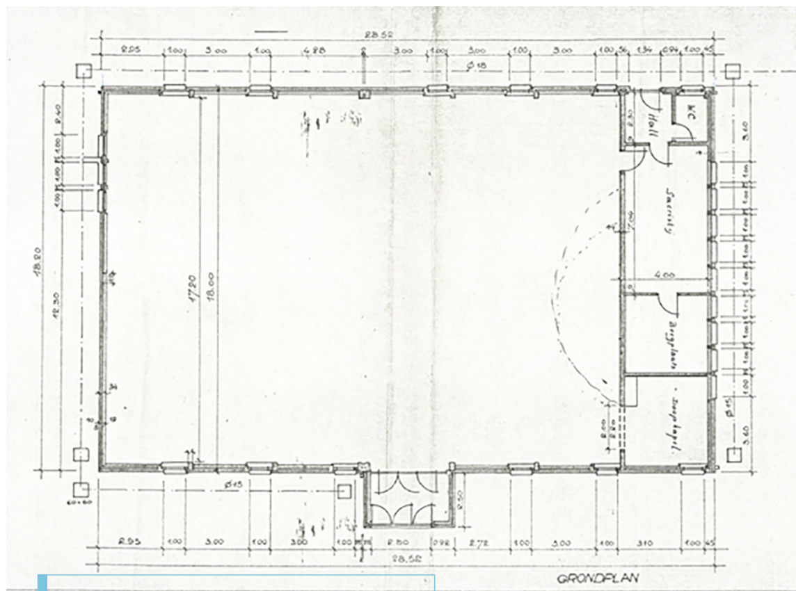
Figuur 16: grondplan van de Onze-Lieve-Vrouwerk
