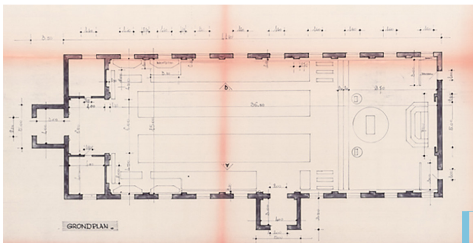
Figuur 3: grondplan van de Sint-Valentinuskerk
